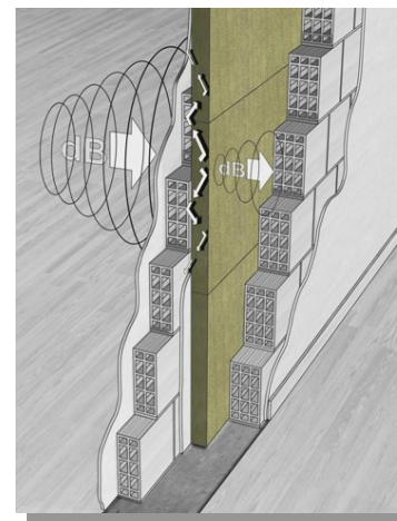
Figura 7. Abbattimento acustico
