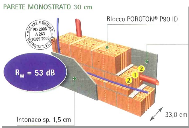
Figura 3. Stratigrafia muratura sp. 33cm
